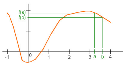
Fonction décroissante sur l'intervalle [3, 4] : si a < b , alors f(a) > f(b) .
